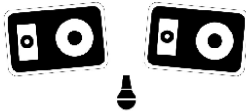
Voc / Git
